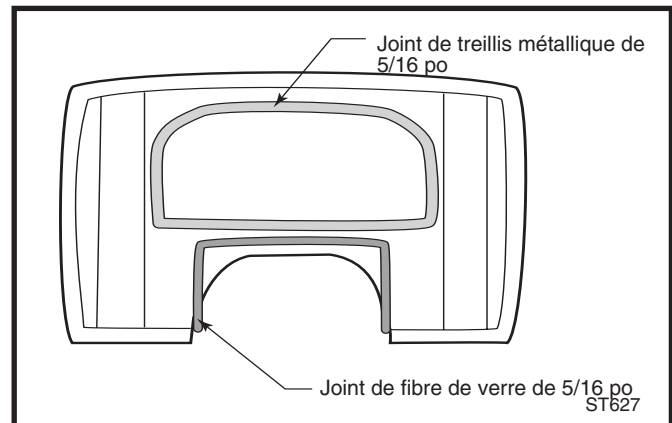
Fig. 40 Un joint de treillis métallique de 5/16 po de pouce scelle la plaque chauffante au dessus du po le. La buse est scellée par un joint de fibre de verre de 5/16 de pouce.
