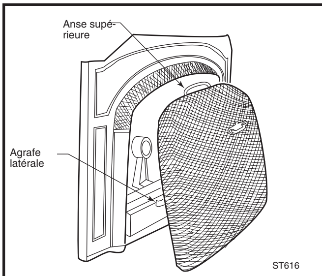
Fig. 32 Inclinez le pare-étincelles pour loger la partie supérieure, puis poussez le bas de façon à ce que les agrafes s'enclenchent.
