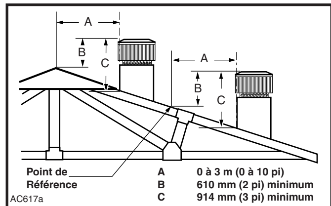
Fig. 2 La règle de 2 -3 et 10 pi pour les cheminées.
