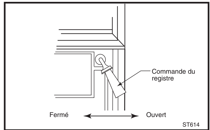
Fig. 30 Lorsque le registre est fermé, la combustion secondaire s'effectue et l'efficacité du poêle Resolute Acclaim est à son maximum.
