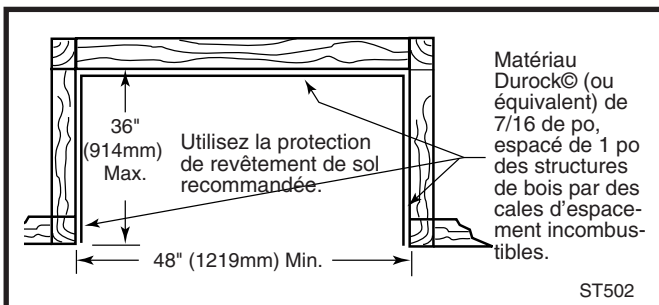
Fig. 24 Plan du sol. Du placoplâtre sur le devant avant se joint au revêtement de l'alcôve en Durock® (ou équivalent).
