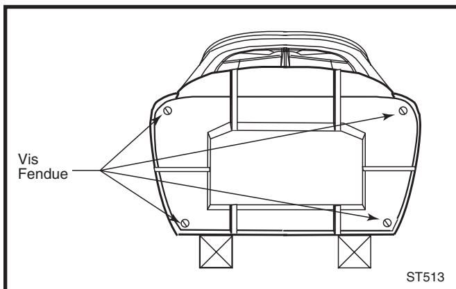
Fig. 27 Enlevez les vis fendues de la partie inférieure du poêle.
