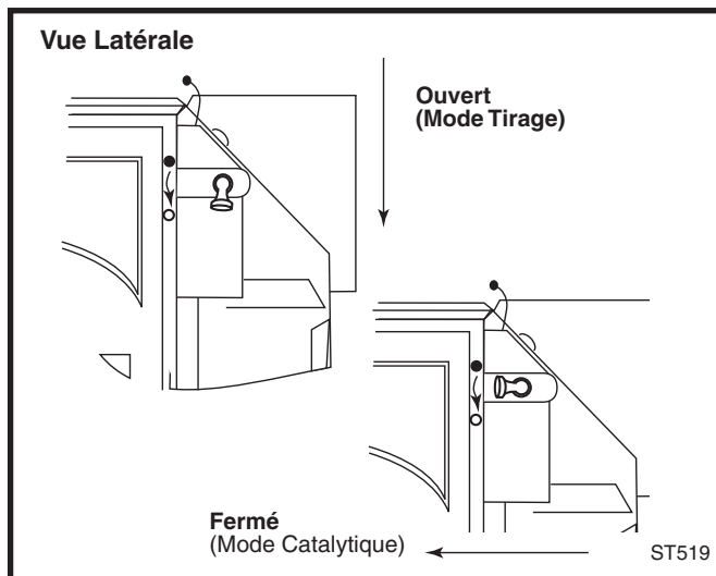
Fig. 34 Le clapet est ouvert ou fermé. Il n'existe aucune position intermédiaire.
