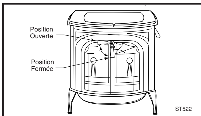
Fig. 37 Pour ouvrir les portes avant, tournez la poignée vers la droite.
