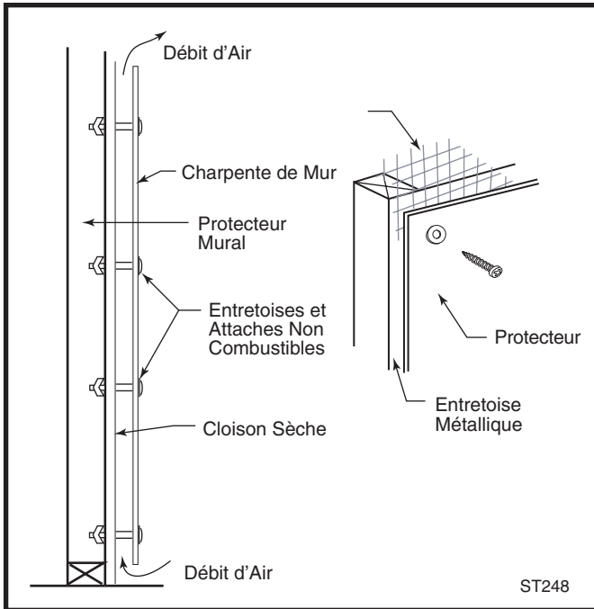
Fig. 13 Construction avec protecteur mural approuvé.
