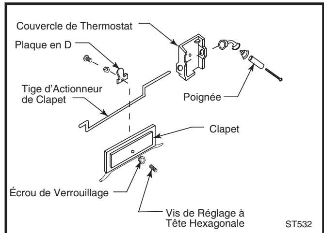
Fig. 45 Serrez la vis de réglage du clapet pour assurer un ajustement serré.
