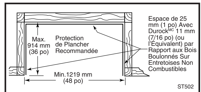
Fig. 16 Plan de plancher avec alcôve. Panneau mural sur la face avant s'aboute au Durock MC (ou l'équivalent) au-dessus du revêtement.
