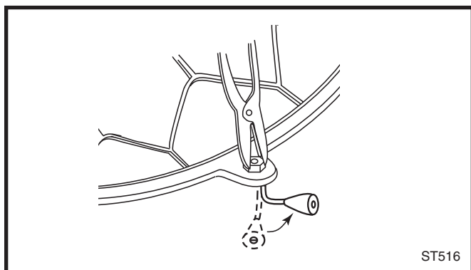
Fig. 31 Fixation de la poignée de la plaque.
