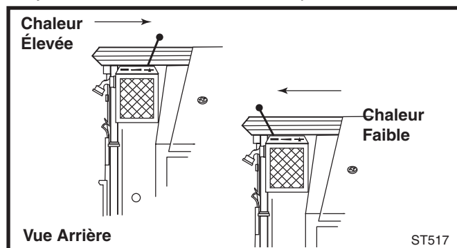
Fig. 33 La poignée du thermostat peut être placée n'importe où entre deux extrêmes pour différents niveaux de chaleur.
