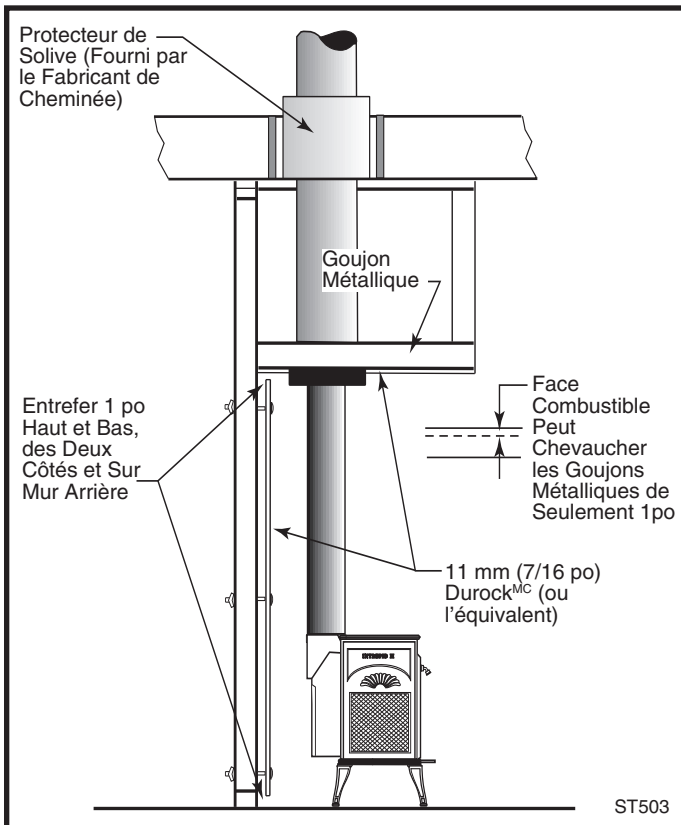
Fig. 17 Section du côté alcôve.
