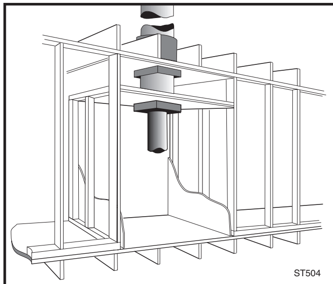
Fig. 18 Vue en coupe de l'installation d'une alcôve.
