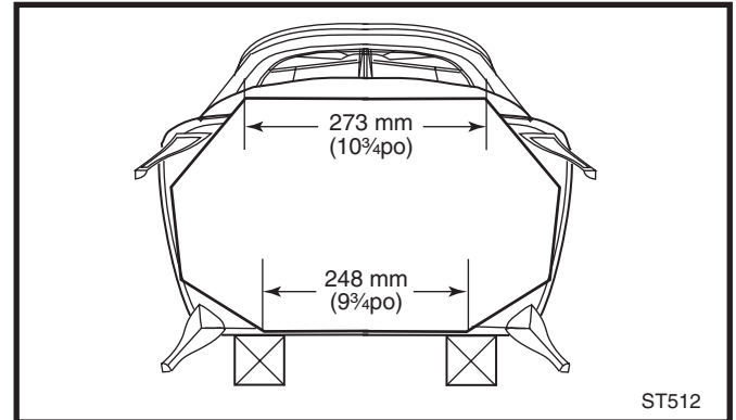
Fig. 28 Fixez l'écran thermique inférieur.
