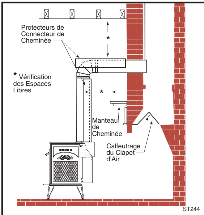
Fig. 7 Le connecteur de cheminée entre dans la cheminée au-dessus du foyer.
