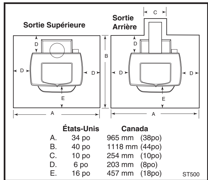
Fig. 11 Dimensions requises pour un protecteur de plancher.
