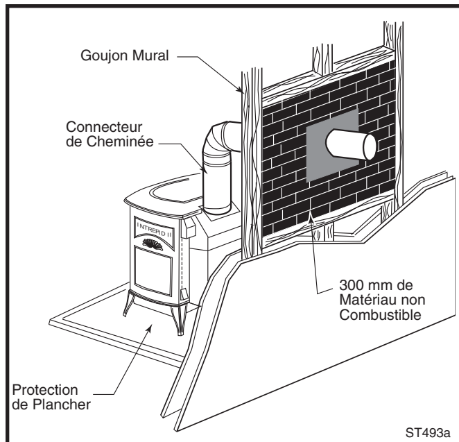
Fig. 9 Un passe-plats de mur approuvé pour les États-Unis.
