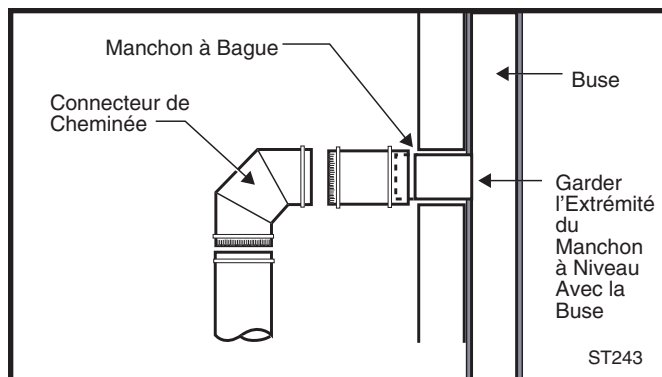
Fig. 5 Le manchon, fait de céramique ou de métal, doit être cimenté solidement en place.
