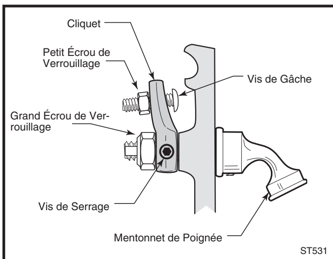
Fig. 44 Tournez la vis de gâche du loquet de porte vers l'intérieur ou l'extérieur pour la serrer ou la desserrer.
