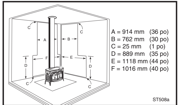
Fig. 24 Installation parallèle, connecteur vertical de cheminée avec poêle, connecteur et protecteurs muraux. Réduction maximale pour murs arrière et latéraux. Les protecteurs muraux peuvent se rejoindre dans un angle. Un écran thermique ayant un diamètre de 610mm (24po) suspendu à 25mm (1po) sous le plafond doit entourer la cheminée.
