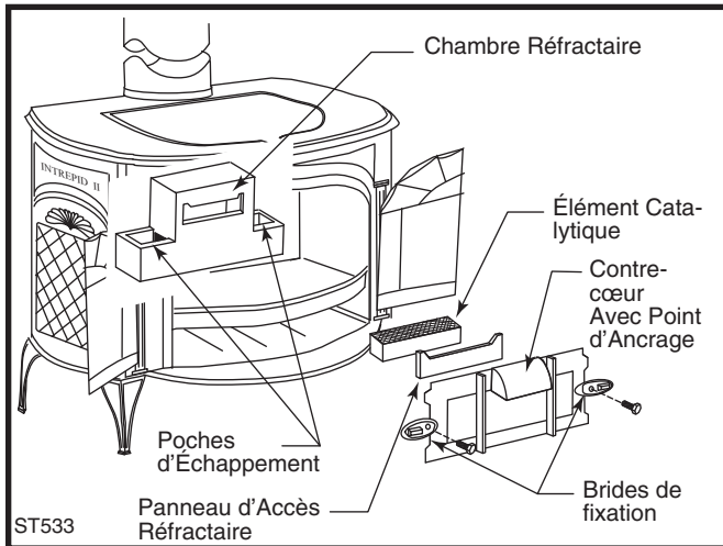
Fig. 46 Dépose de l'élément catalytique.
