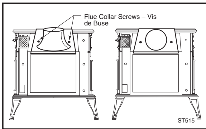
Fig. 30 Inversion de la buse.
