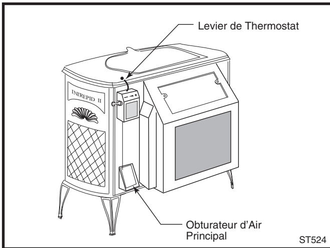
Fig. 43 L'obturbateur d'air principal doit pouvoir se déplacer librement.
