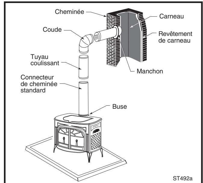
Fig. 6 Connexion de cheminée dans une installation autonome.
