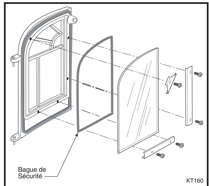
Fig. 42 Installation de la vitre de porte.
